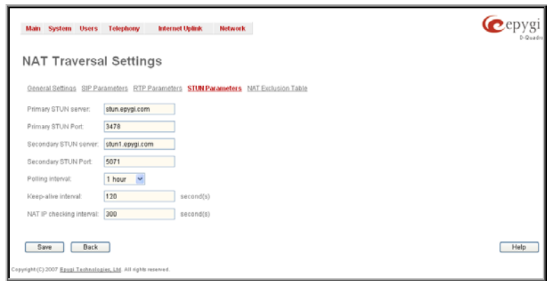
Fig. II-119: STUN Parameters page
